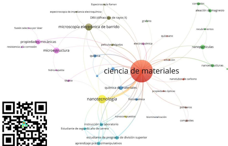
Fig. 4. Red de co-ocurrencia, resumen de artículos de 2003 a 2024. Método de análisis de redes, algoritmo de agrupamiento de Louvan, fuerza de repulsión 0.1, número mínimo de aristas 2.
