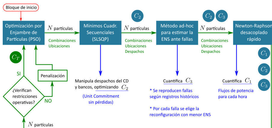
FIGURA 1 Diagrama de bloques del método híbrido implementado.
