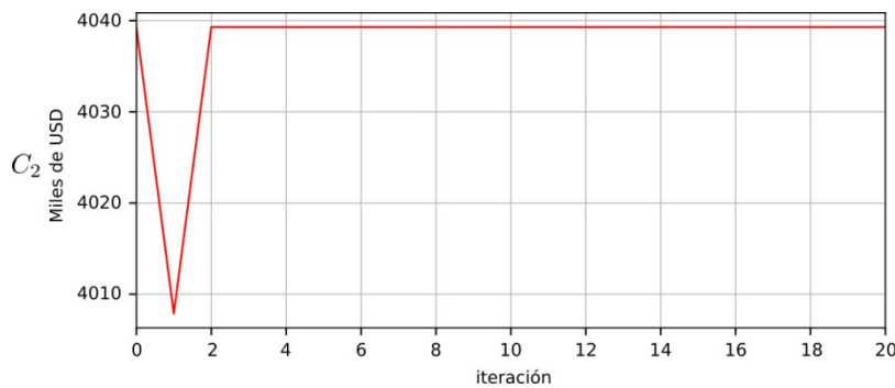
FIGURA 6 Evolución iterativa del costo anual de O&M del sistema ( C_2 ).
