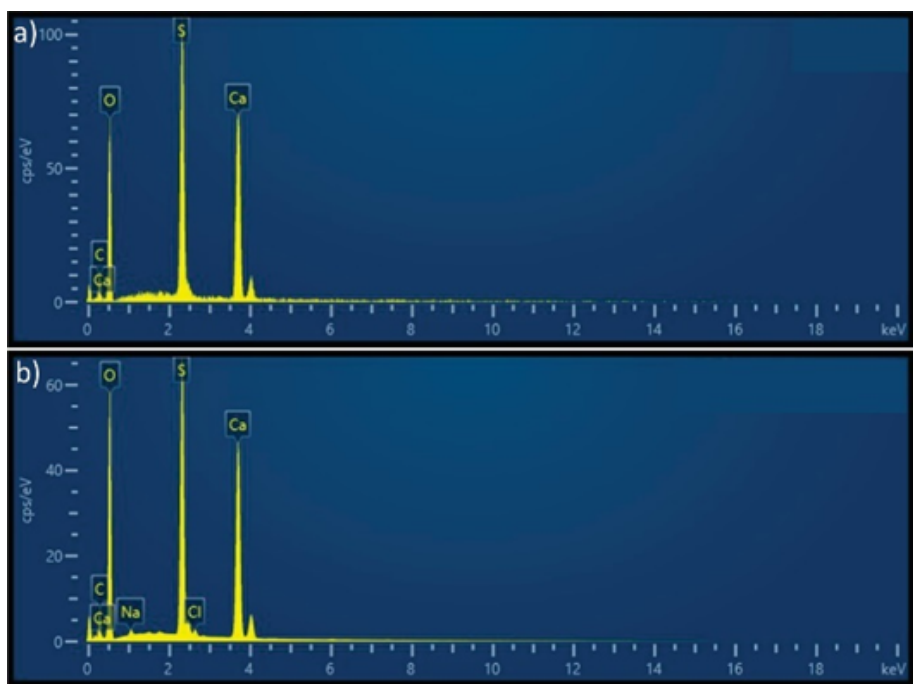
FIGURA 8 Espectros composicionales promedio de los puntos 1, 2 y 3 de los cristales, a) tabular y b) columnar, obtenidos mediante análisis EDX.
